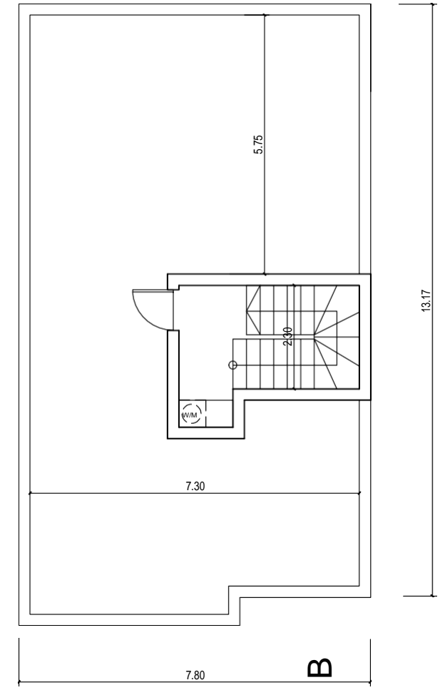
ΚΑΤΩΦΗ ΟΡΟΦΗΣ
