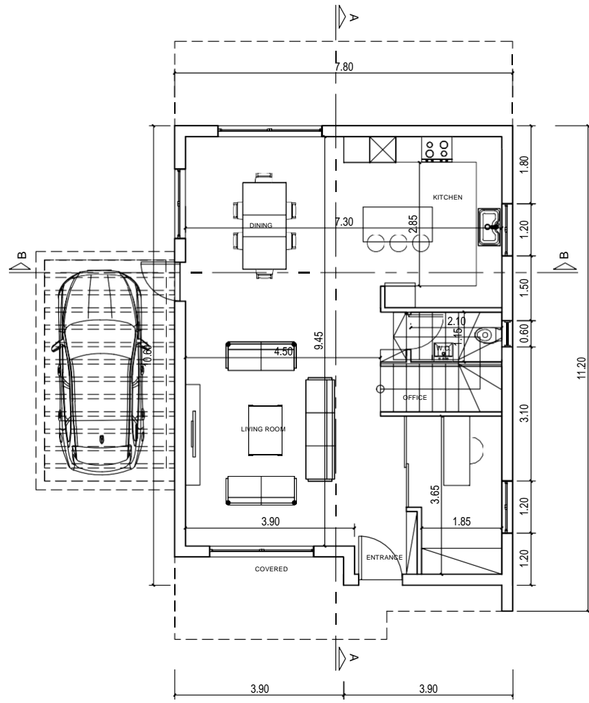
ΚΑΤΩΦΗ ΙΣΟΓΕΙΟΥ
