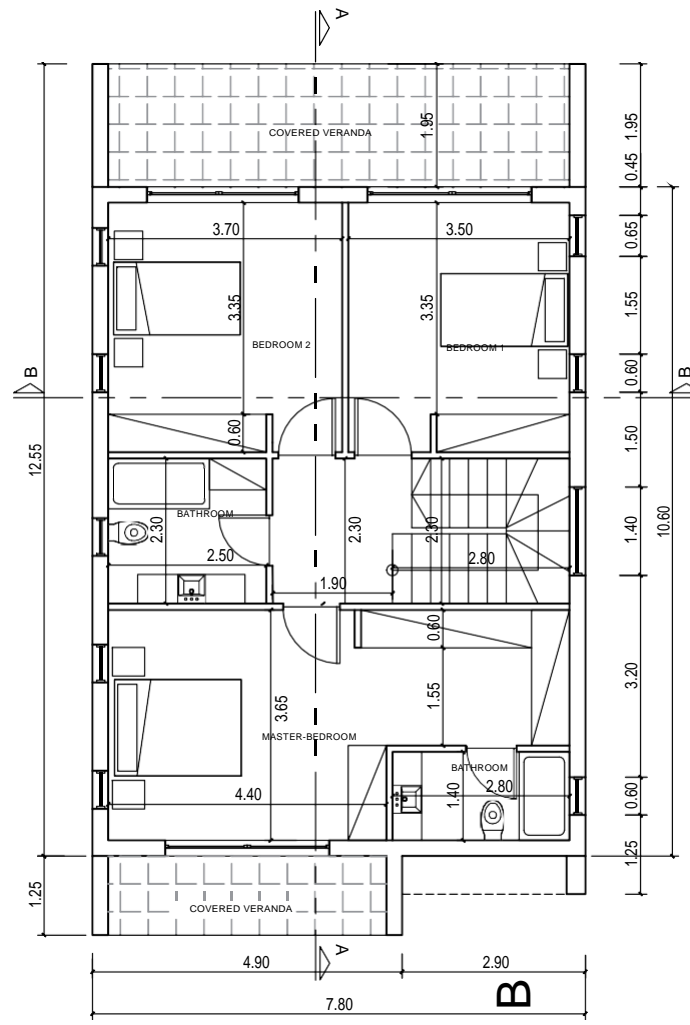
ΚΑΤΩΦΗ ΟΡΟΦΟΥ
